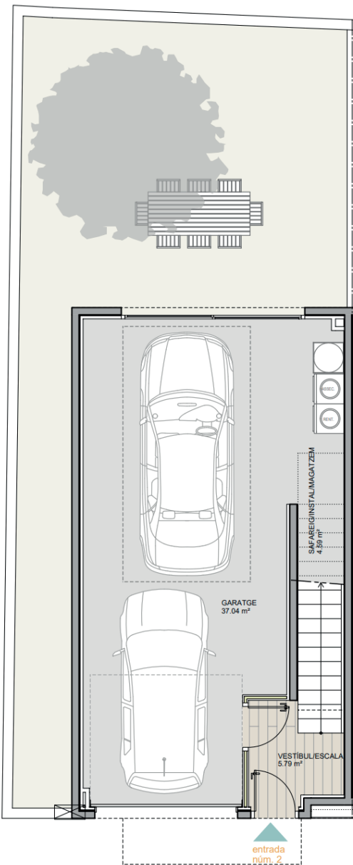
PLANTA BAIXA E: 1/75
