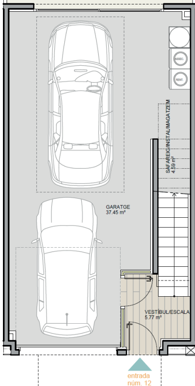
PLANTA BAIXA E: 1/75
